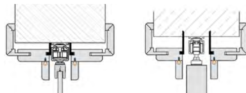
Deckenmontage unter Sturz
