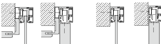
Montage ohne DUFU
