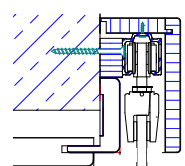
Montage mit Schiebetürfutter für Glastür
