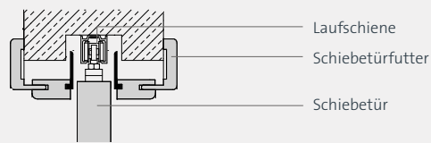
Holzschiebetür im Sturz
