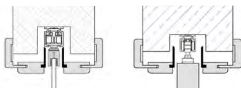
Deckenmontage im Sturz
