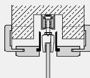
Glasschiebetür im Sturz
