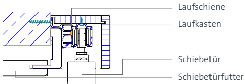
Montage mit Schiebetürfutter für Holztür
